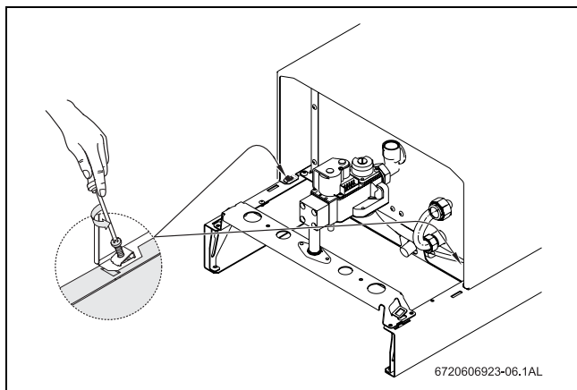
Att. 12 Apvalka noņemšana
