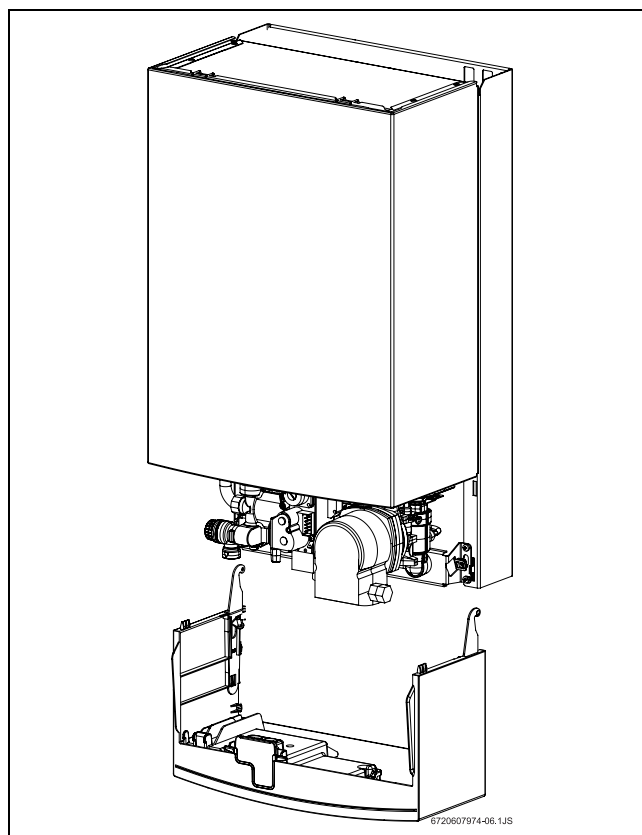
Att. 11 Sadales kārbas noņemšana
