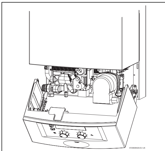
Att. 28 Servisa pozīcija gāzes ieregulēšanai
