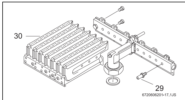
Att. 31 Degļa bloks
