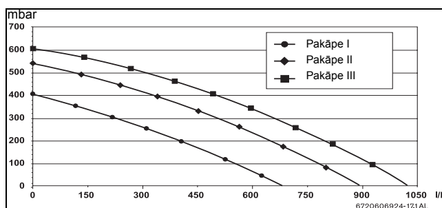
Att. 6 Sūkņa raksturlīkne
