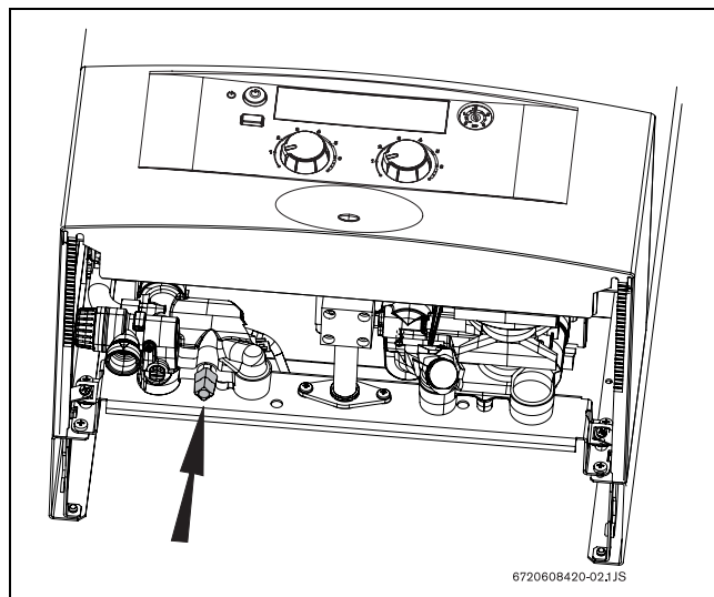
Att. 13 Uzpildes krāns
