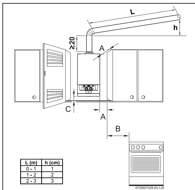
Att. 7 Minimālais attālums
