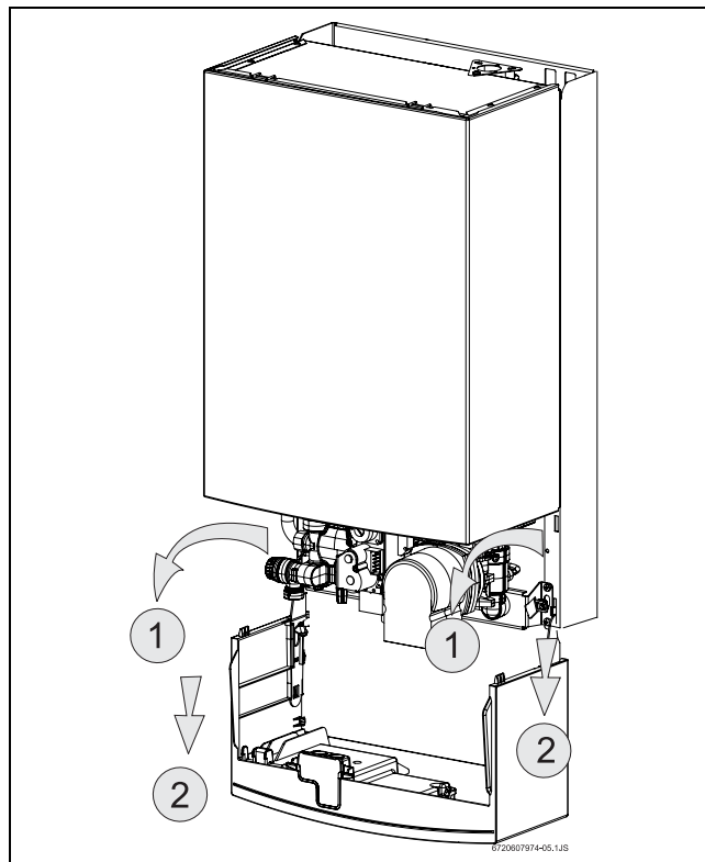
Att. 10 Servisa pozīcija
