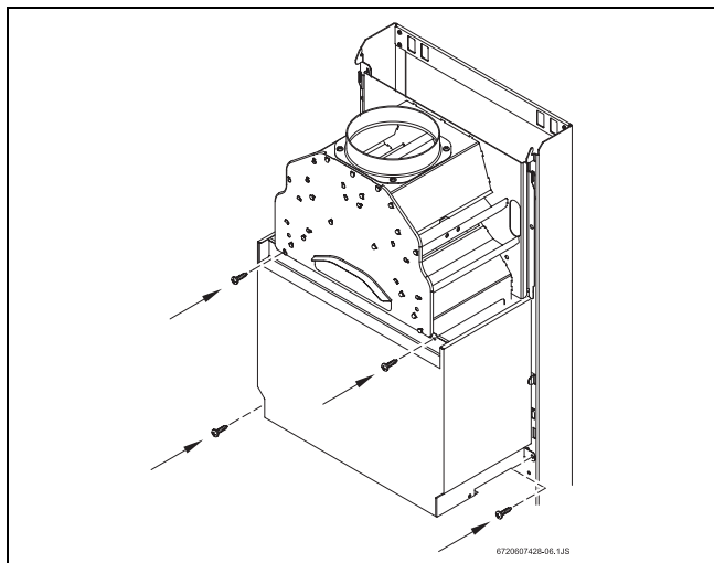
Att. 30 Degkameras priekšējā siena
