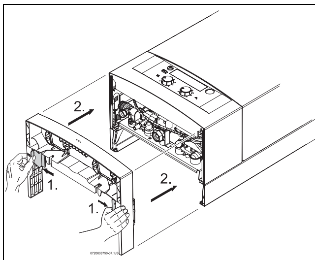
Att. 15 Paneļa novietošana
